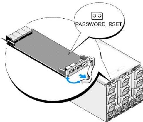
Abbildung 12-1. Kennwort-Reset-Jumperposition
