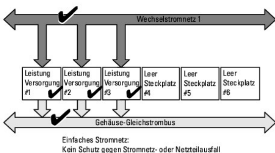
Abbildung 9-3. „Keine Redundanz“ bei drei Netzteilereinheiten im Gehäuse
