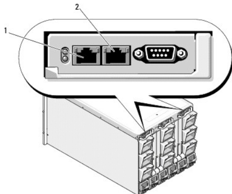
Abbildung 1-1. Dell M1000e-Gehäuse und CMC
